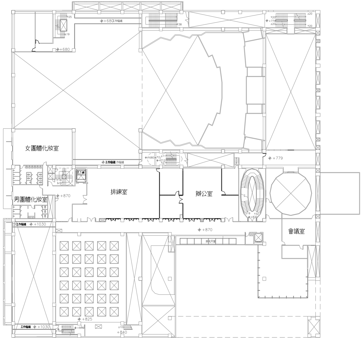
三樓平面圖
