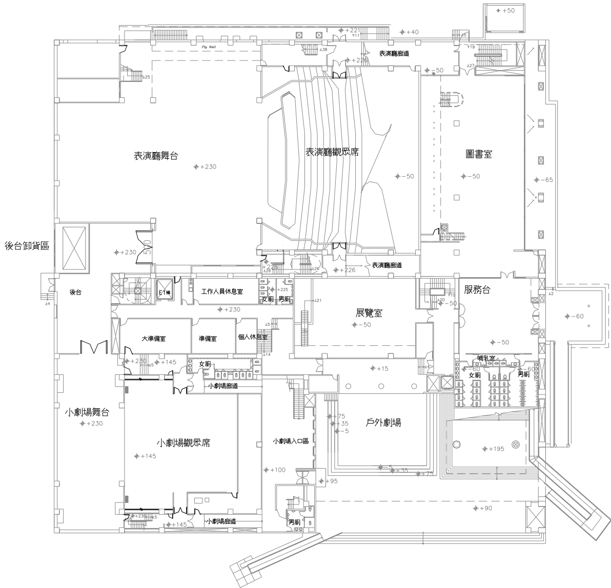
一樓平面圖
