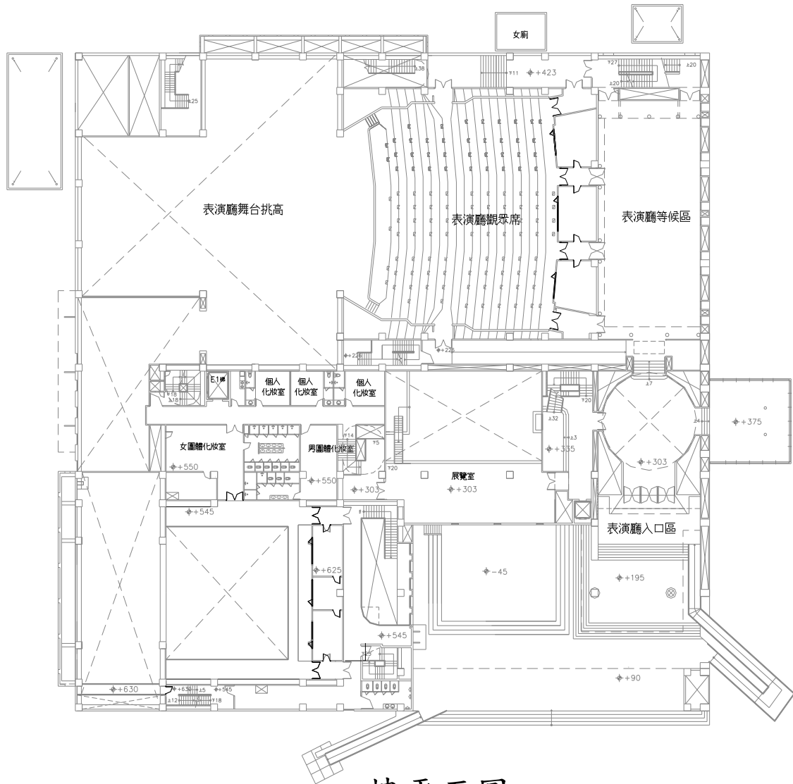
二樓平面圖
