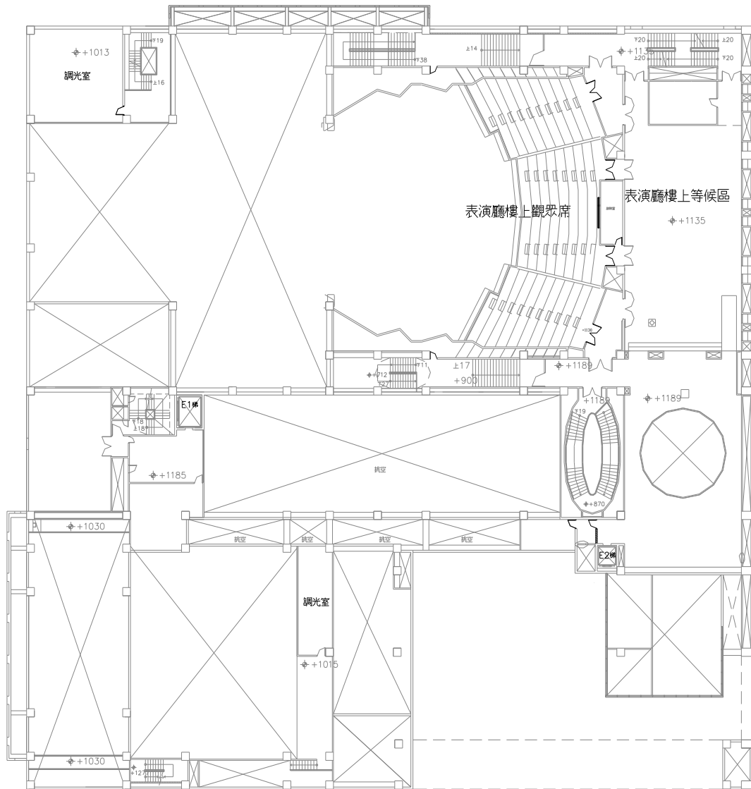
四樓平面圖
