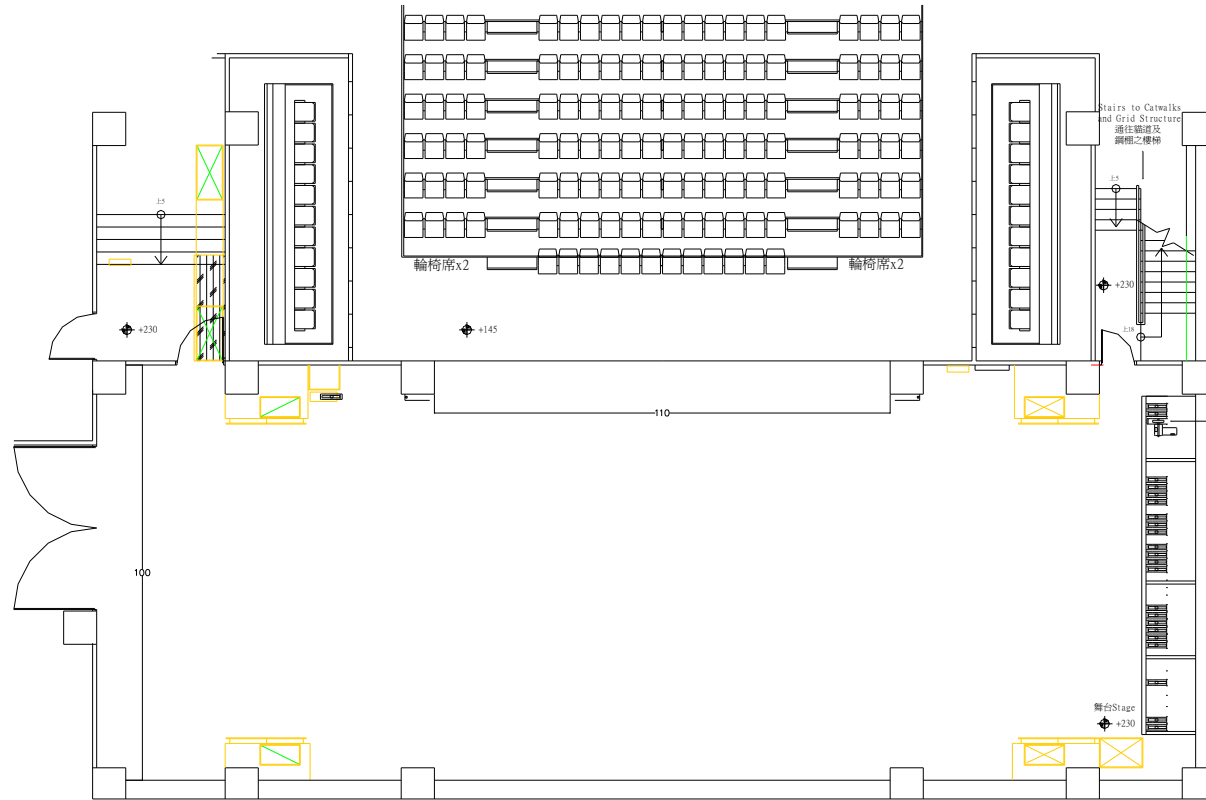
小劇場舞台平面圖
