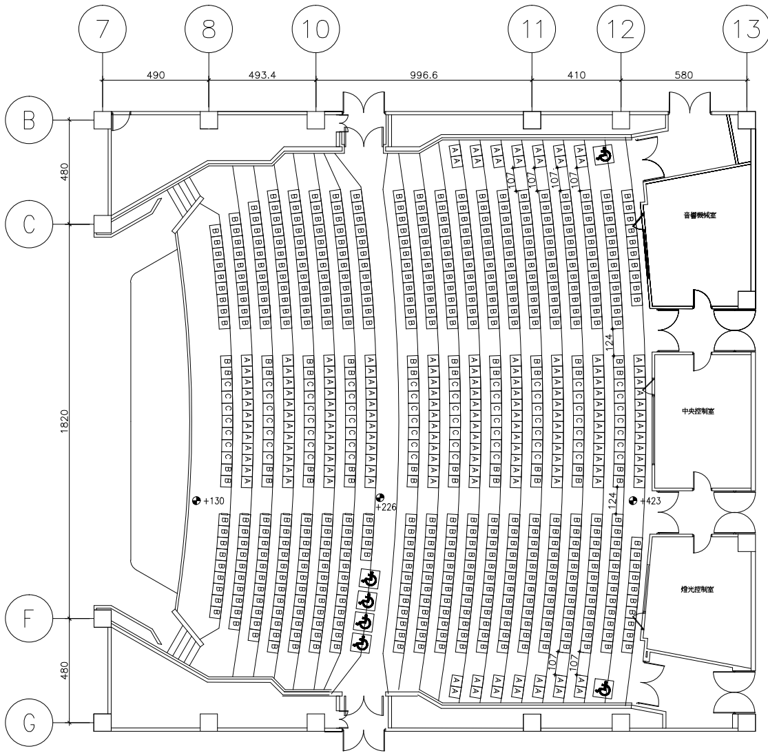
樓下觀眾席座椅平面圖
