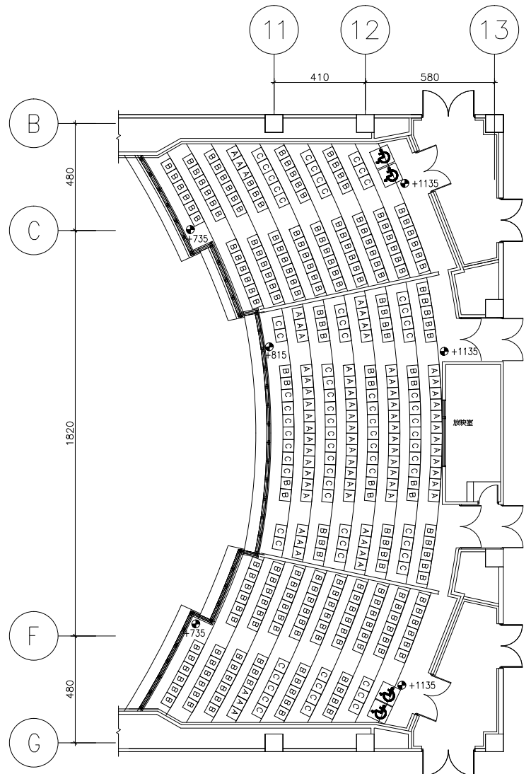
樓上觀眾席座椅平面圖
