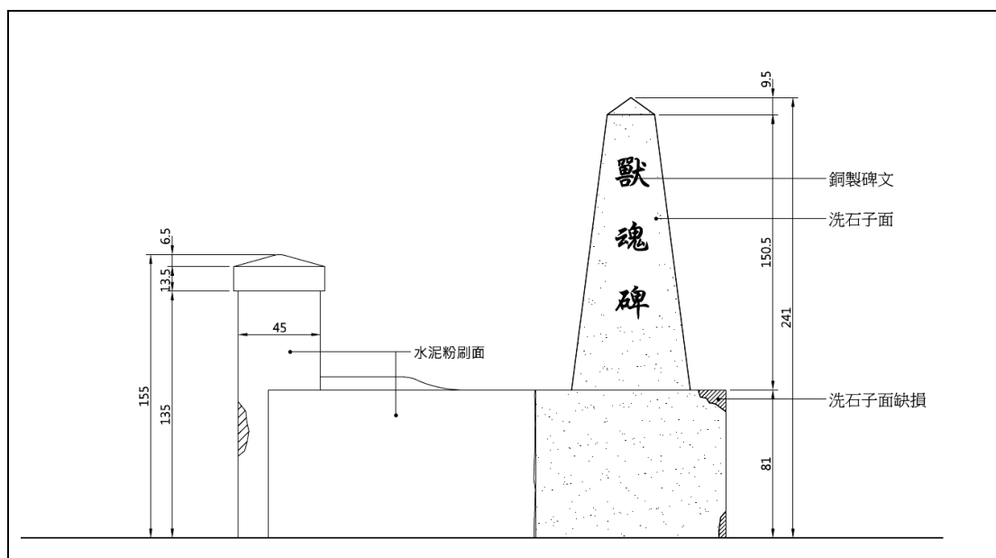
圖表 58：獸魂碑正面損壞調查圖
