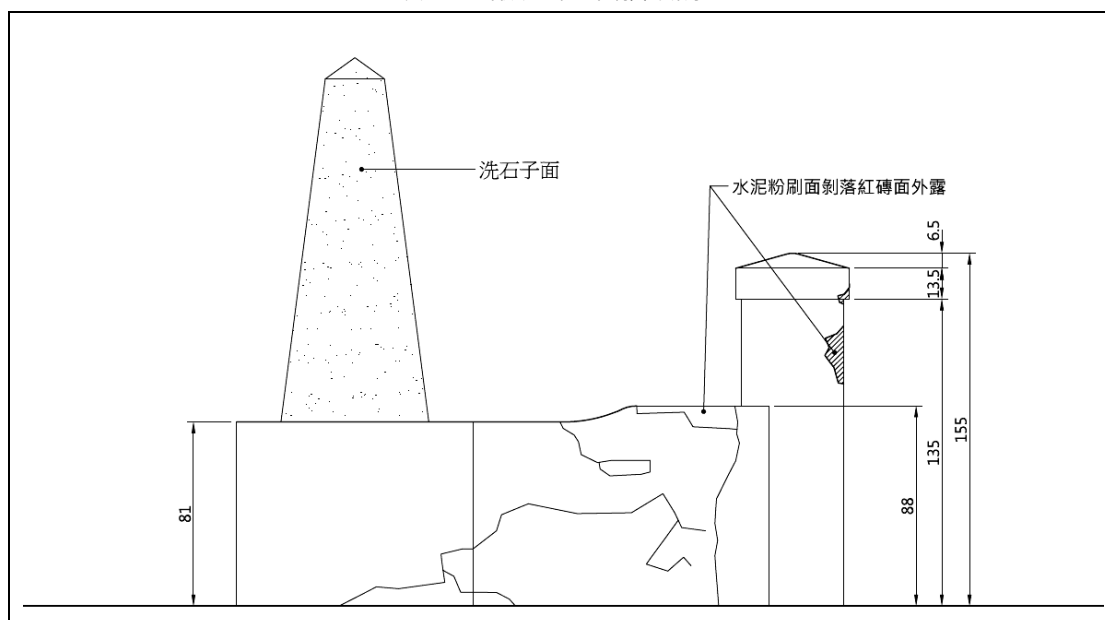
圖表 59：獸魂碑背面損壞調查圖
