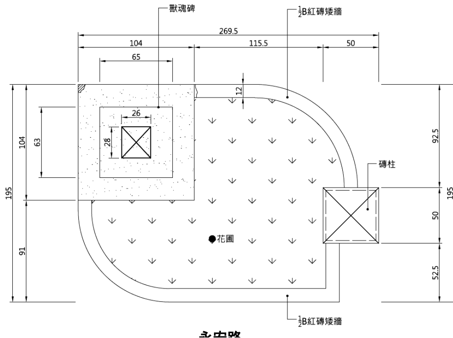
圖表 44：獸魂碑平面圖
